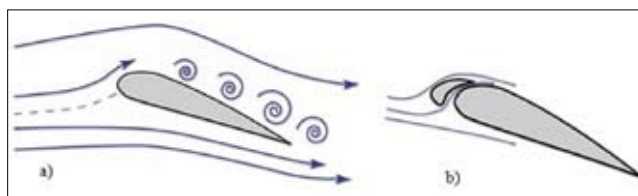
Figura 7. a) profil krahut në kënd të lartë (humbje e forcës ngritëse), b) efekti i fryrjes nëpërmjet slateve
